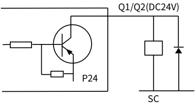
晶体管输出电路
