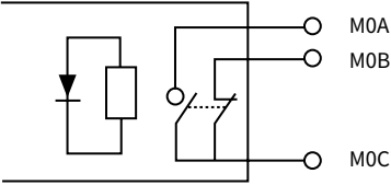
准停到位继电器输出原理图
