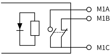
故障继电器输出原理图
