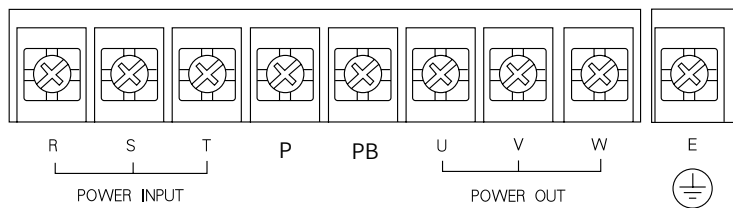
1.5~75A和220~320A主回路端子结构
