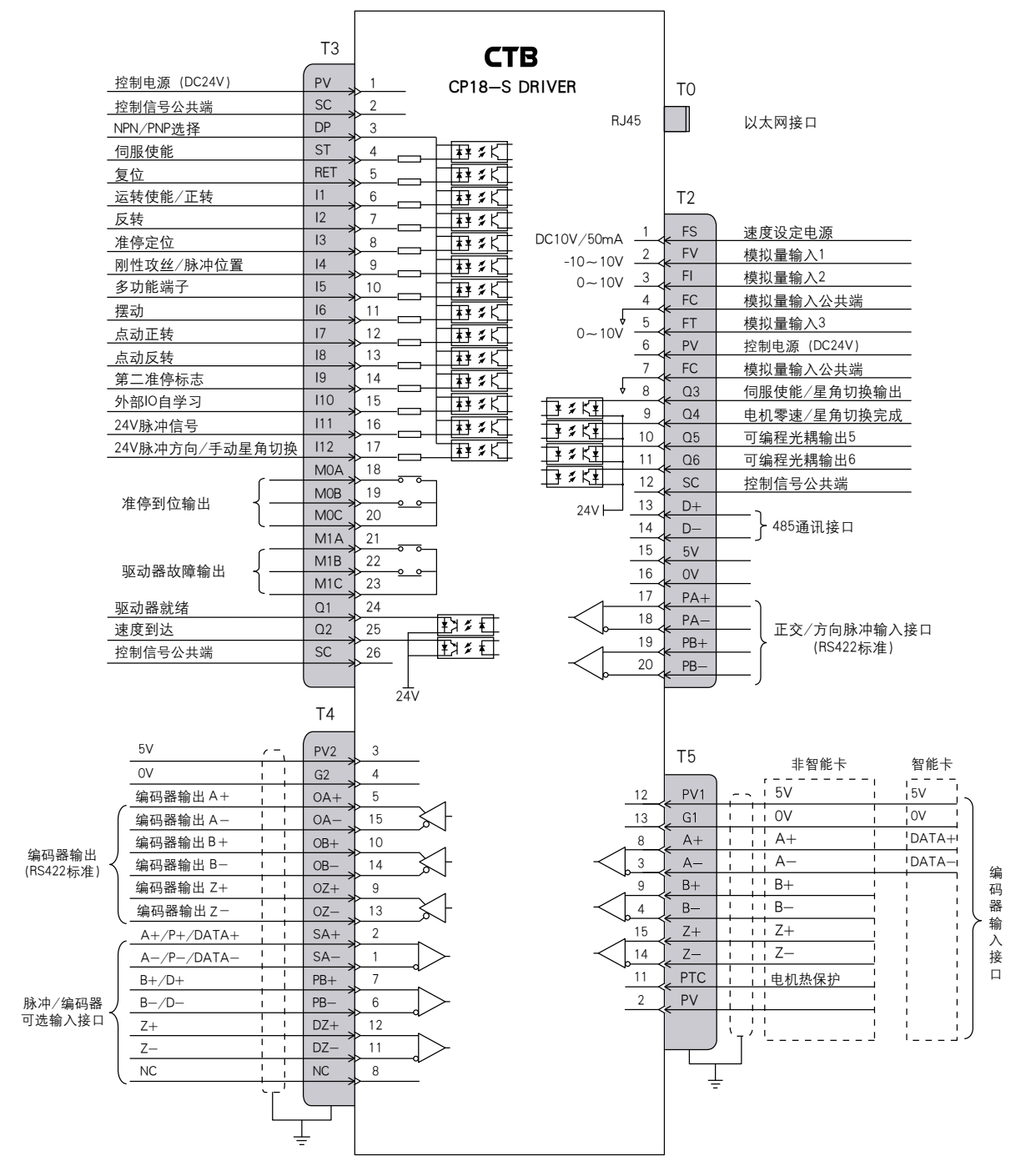
D18-S 控制接线图
