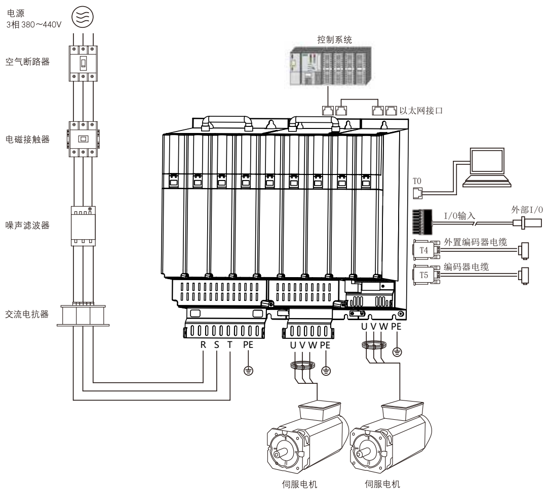
驱动器与周边器件连接示意图
