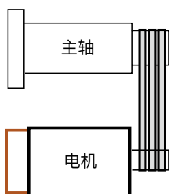
直连结构图
