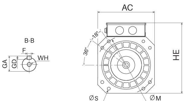
Z18BF-Z18BH 机座
