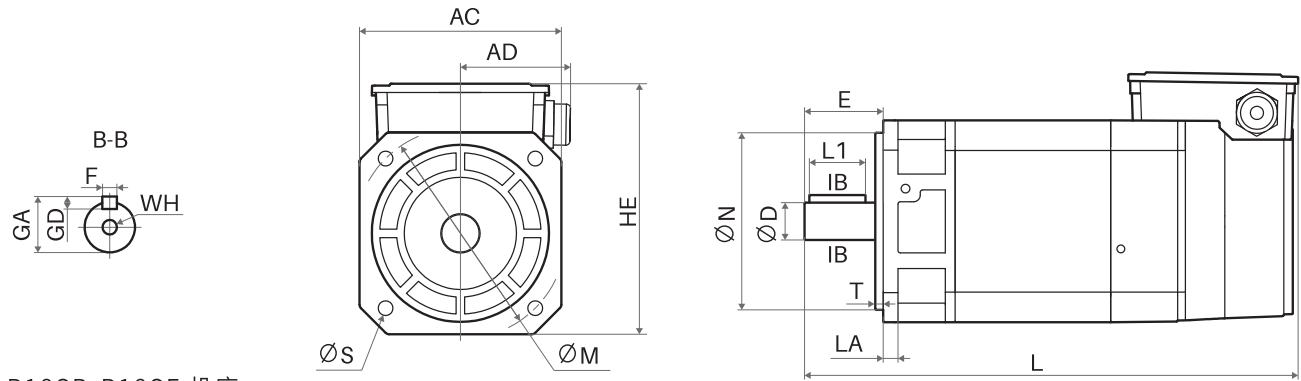
P18SB-P18SE 机座
