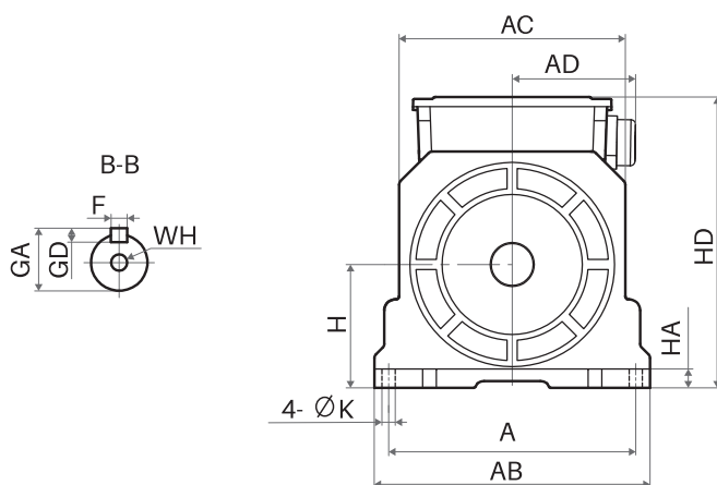
Z18A-Z18H 机座
