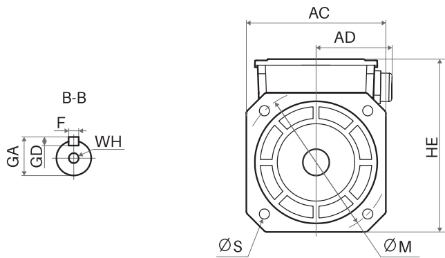
P18SB-P18SE 机座
