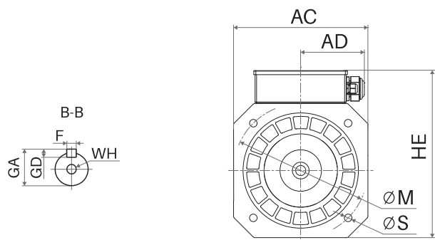
Z18BA-Z18BE 机座
