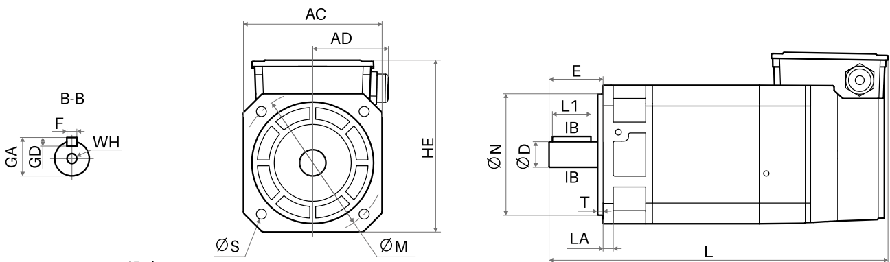
P18SB-P18SE 机座
