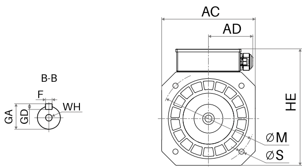
Z18BA-Z18BE 机座
