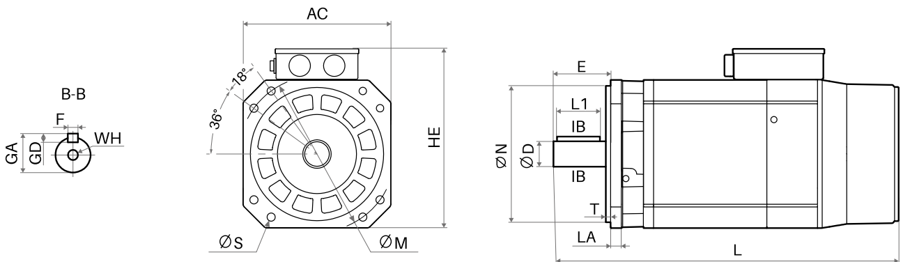
P18SF-P18SH 机座
