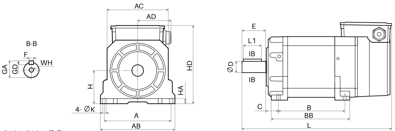
Z18A-Z18H 机座
