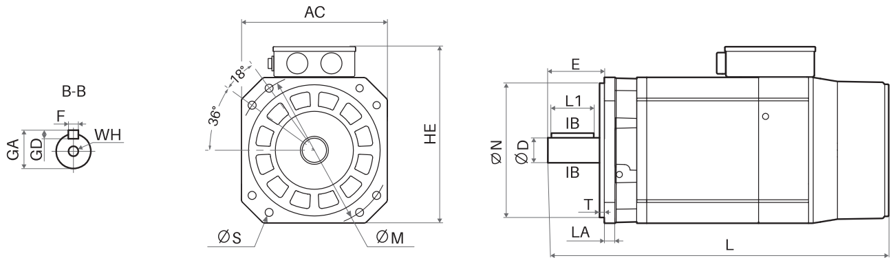
P18SF-P18SH 机座
