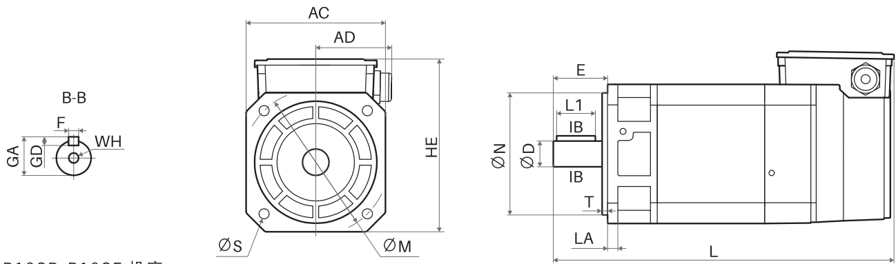
P18SB-P18SE 机座
