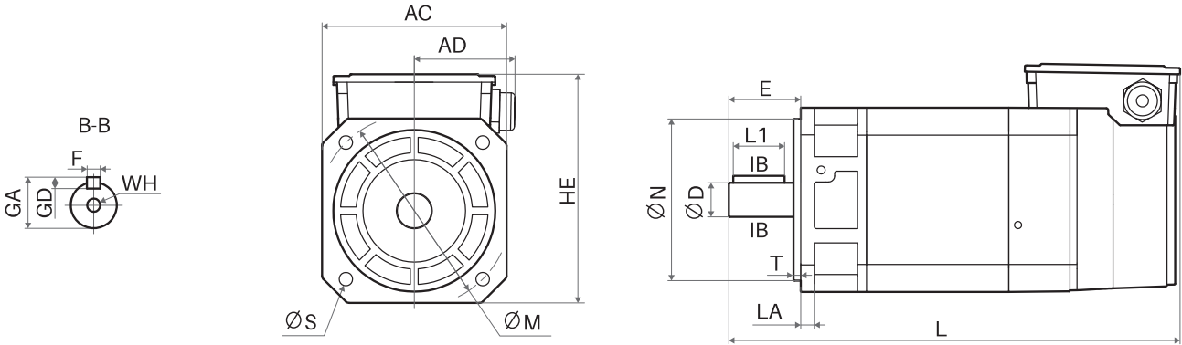
Z18PB、Z18PC、Z18PE 机座
