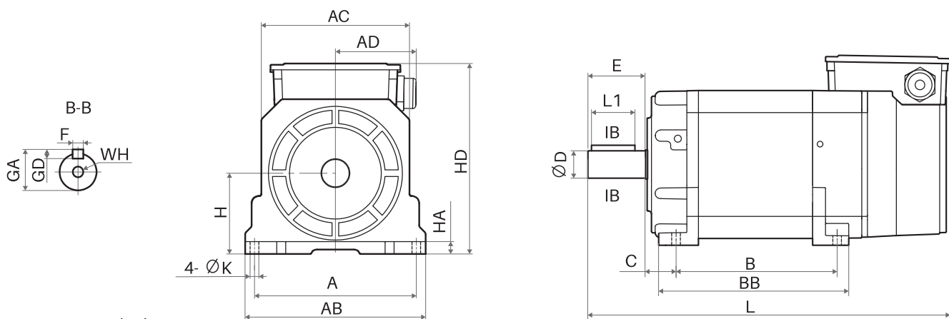
Z18A-Z18H 机座
