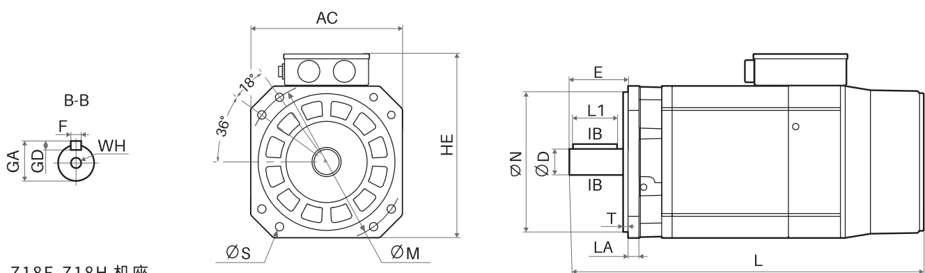
Z18F-Z18H 机座
